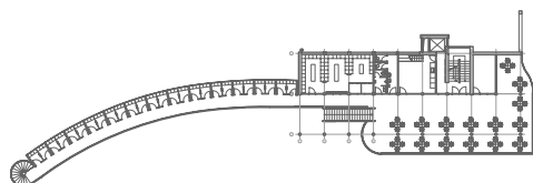
Pôdorys 2. np
